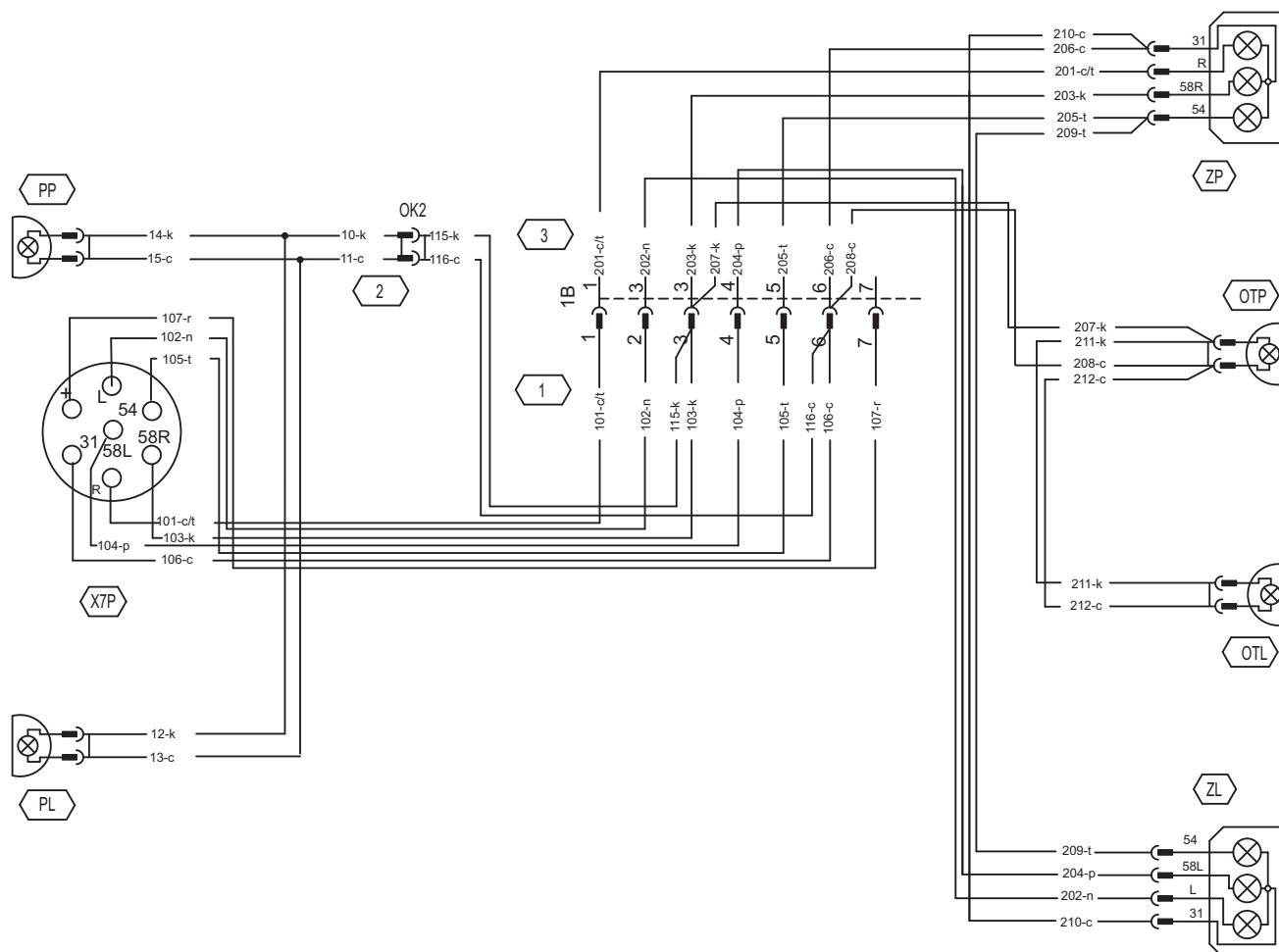
RYSUNEK 3.12 Schemat ideowy instalacji elektrycznej
