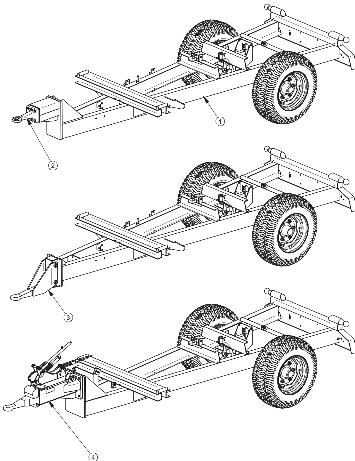
RYСУNEK 3.2 Wersje ramy dolnej
