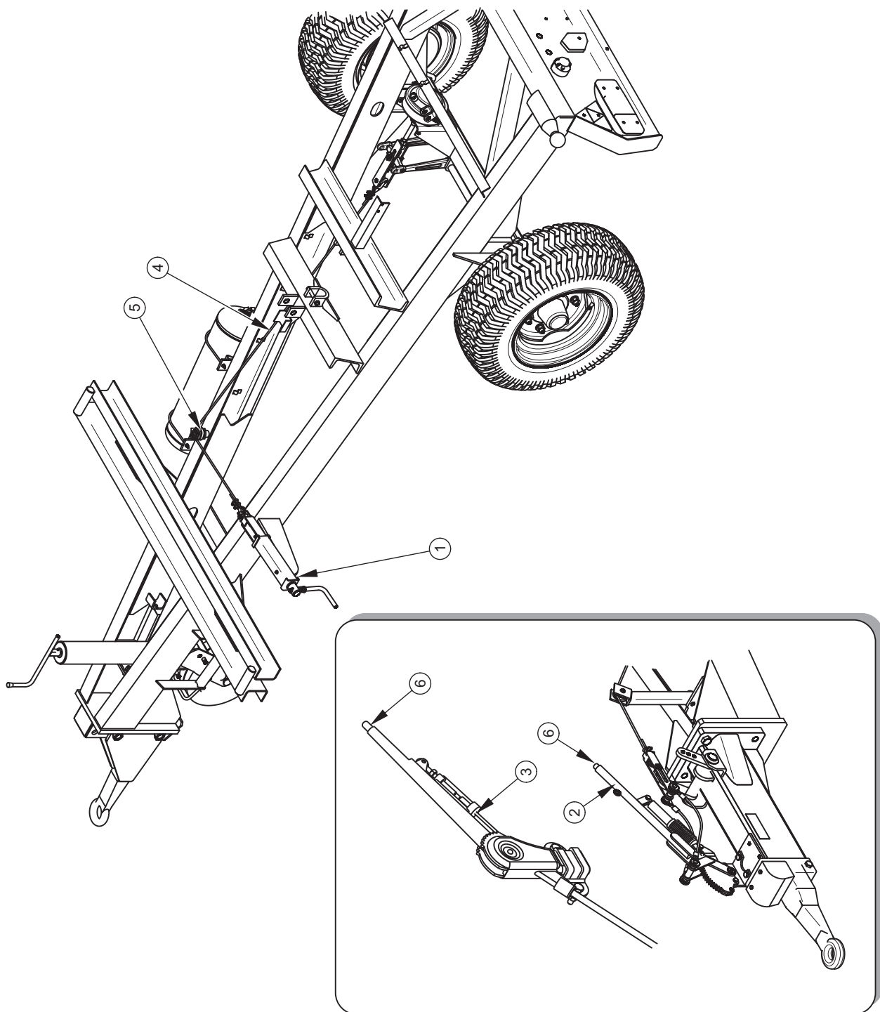
RYSUNEK 3.11 Budowa hamulca postojowego z mechanizmem korbowym
