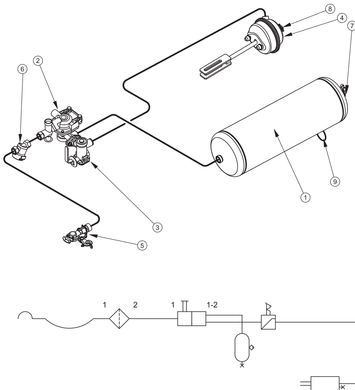
RYSUNEK 3.6 Budowa i schemat instalacji hamulcowej pneumatycznej jedнопrzewodowej
