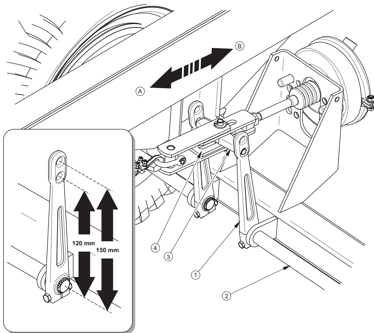
RYСУNEK 5.4 Regulacja hamulców mechanicznych osi jezdnej
